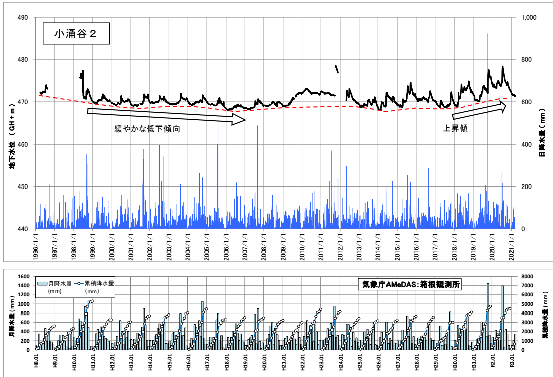
図 3.4-5 地下水位変動グラフ(小涌谷 2)
